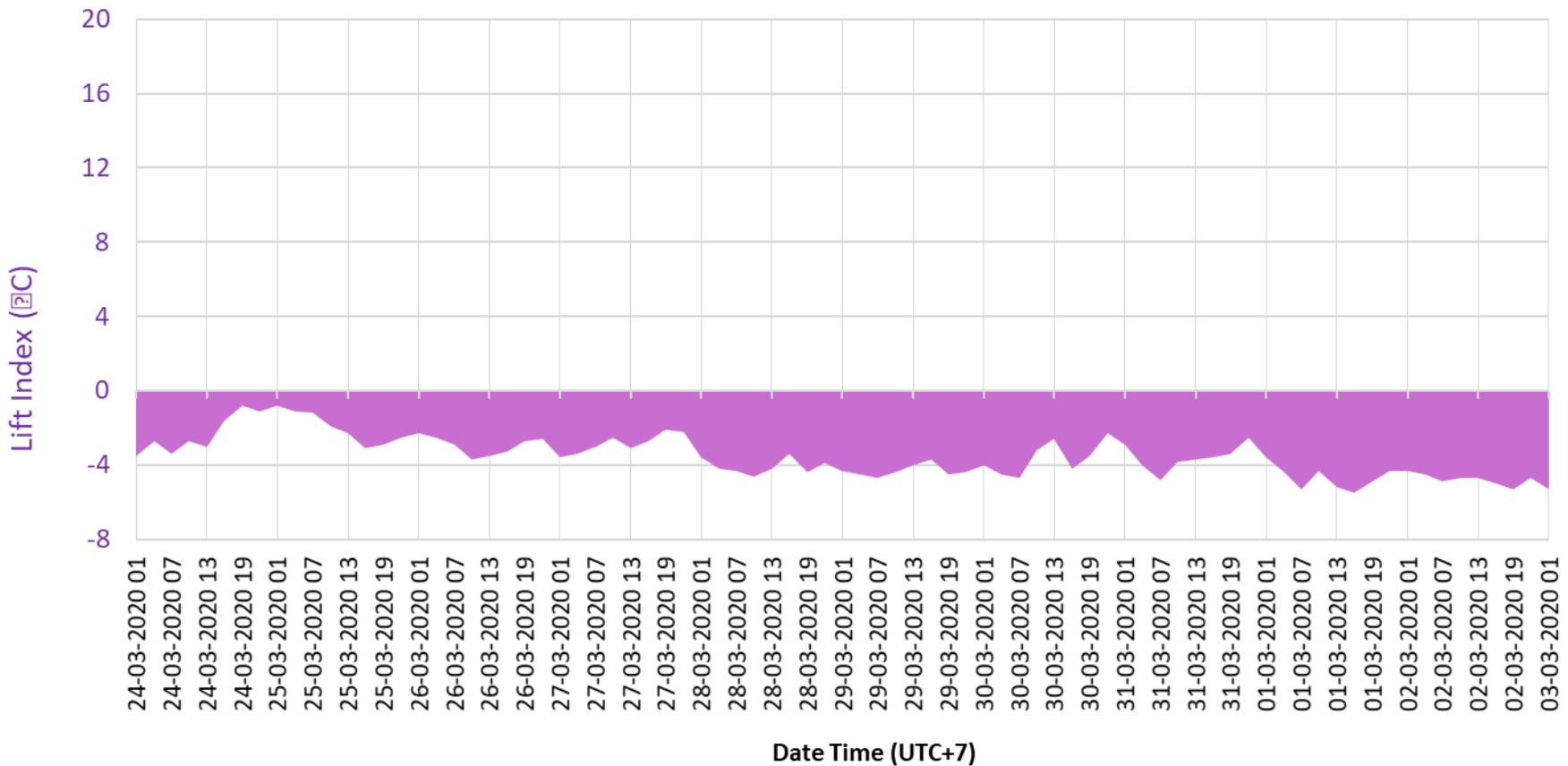
Lift Index (°C)
